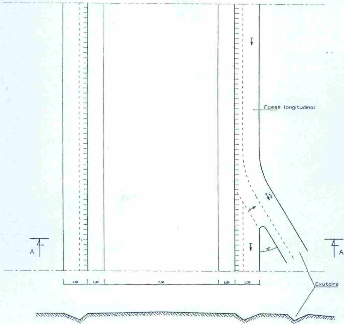
COUPE A-A
